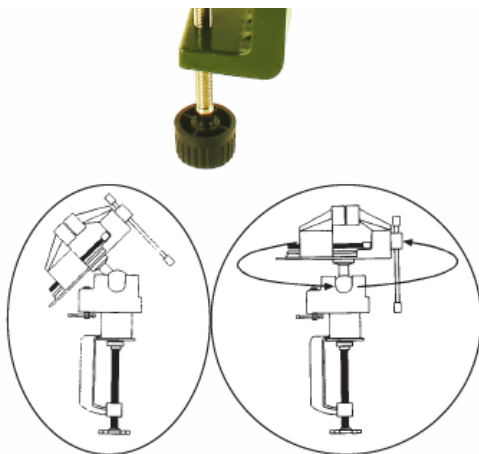
ET-104 Etau ALUMINIUM multi-angles - 75 mm Montage sur tables de 10 à 52 mm Pivotant à 360°. Poids : 2,2 kg MULTI-ANGLE ALUMINIUM VICE - 75 mm Fits 10 to 52 mm thick benches - Pivoting at 360°. Weight : 2.2 kg
